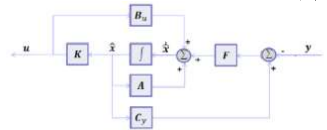
Fig. 3. LQR controller.
